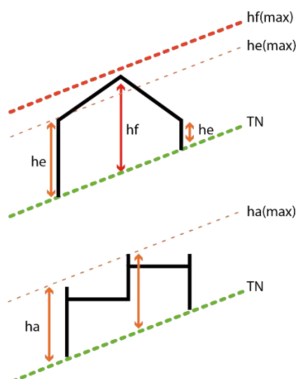
Figure 19 Principe de calcul de la hauteur (avec TN le terrain naturel avant travaux, he la hauteur à l'égout, hf la hauteur au faîtage, ha la hauteur à l'acrotère et h_{max} la hauteur référence du PLUiH)
